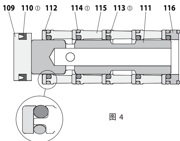
主阀剖视图
